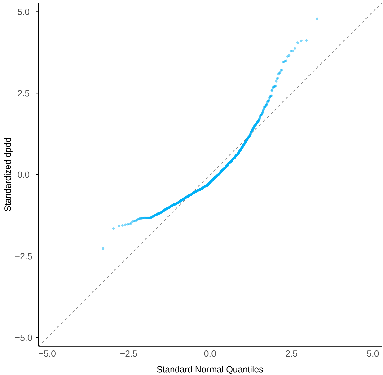
Normal Q-Q: dpdd
